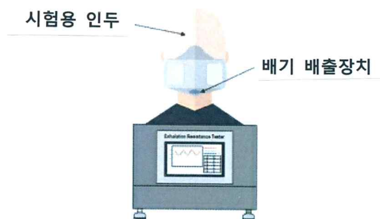
그림 3. 배기 밸브 시험
